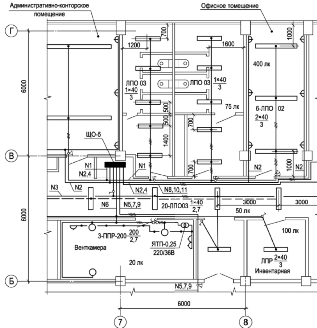
Рисунок Б.1 - Пример оформления плана расположения электрического оборудования и прокладки электрических сетей для производственного здания
